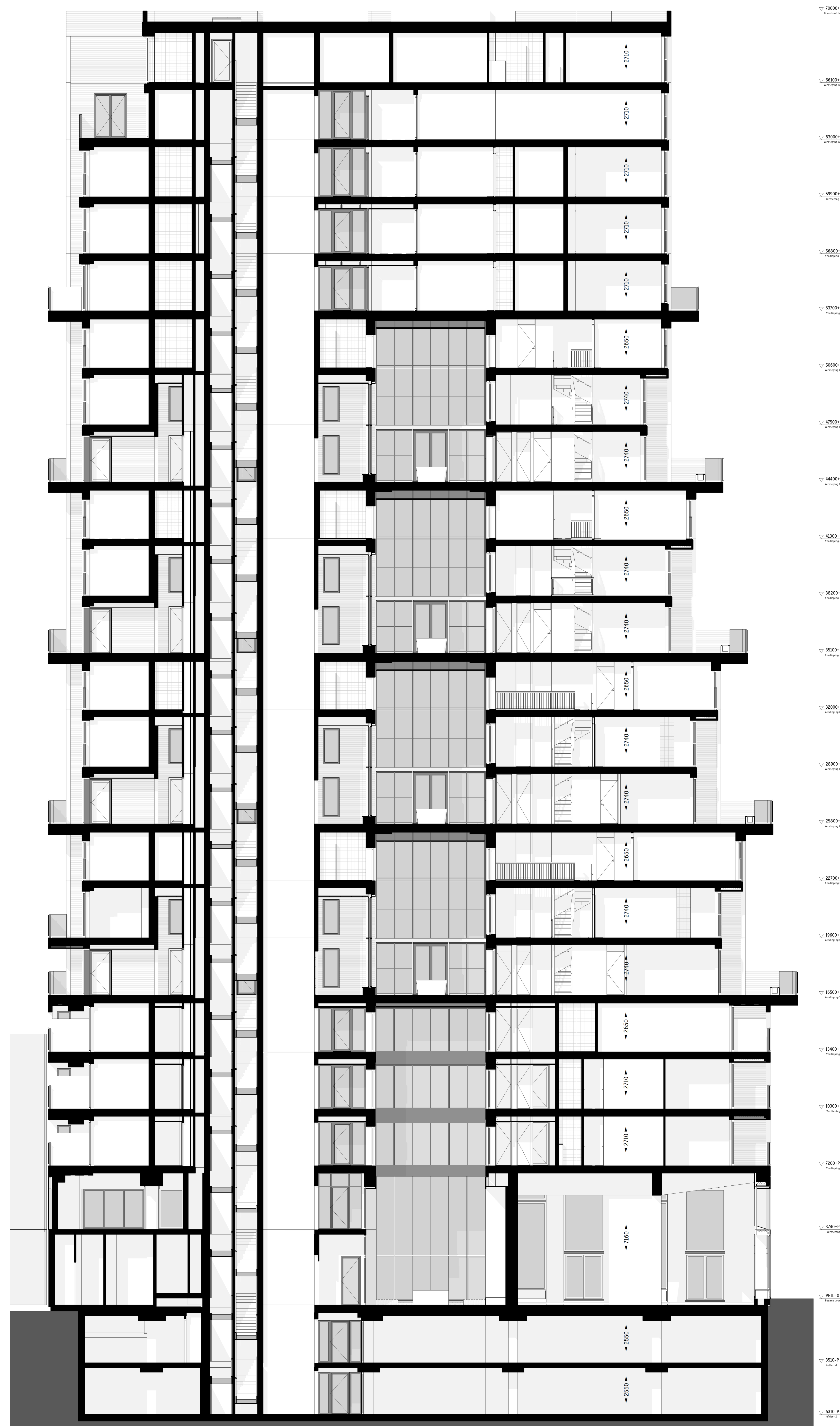
Doorsnede A-A 1:100
