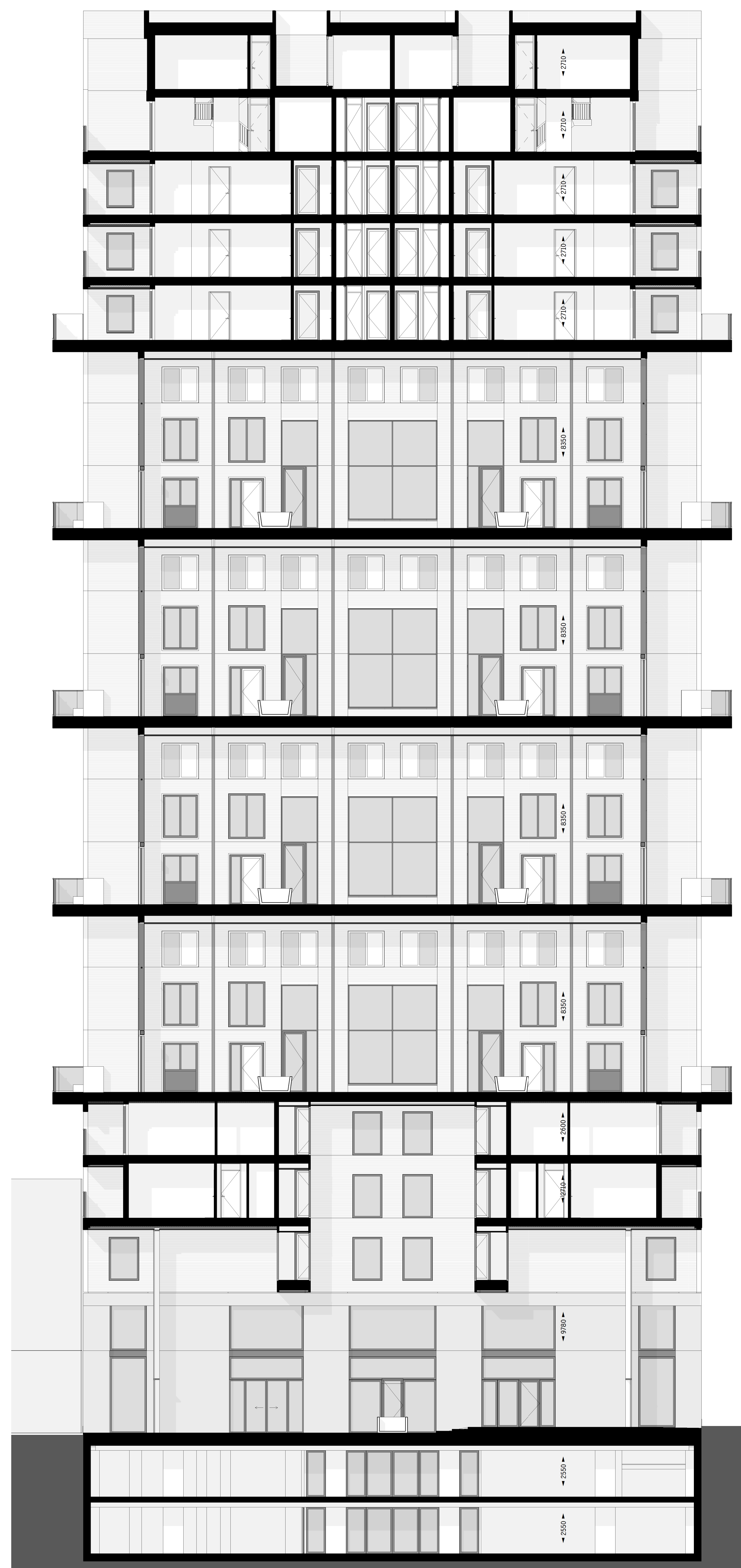
Doorsnede C-C 1:100
