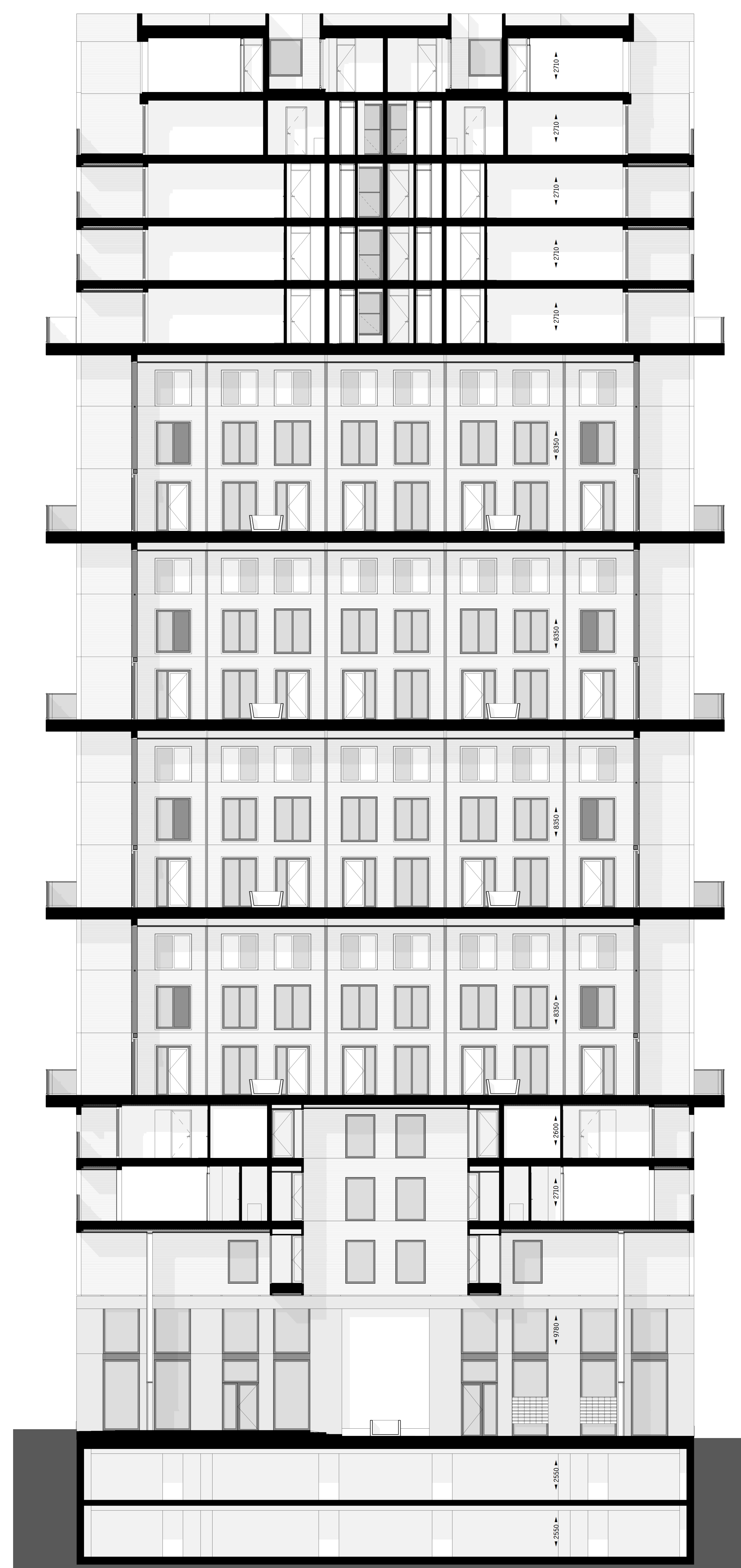
Doorsnede D-D 1:100
