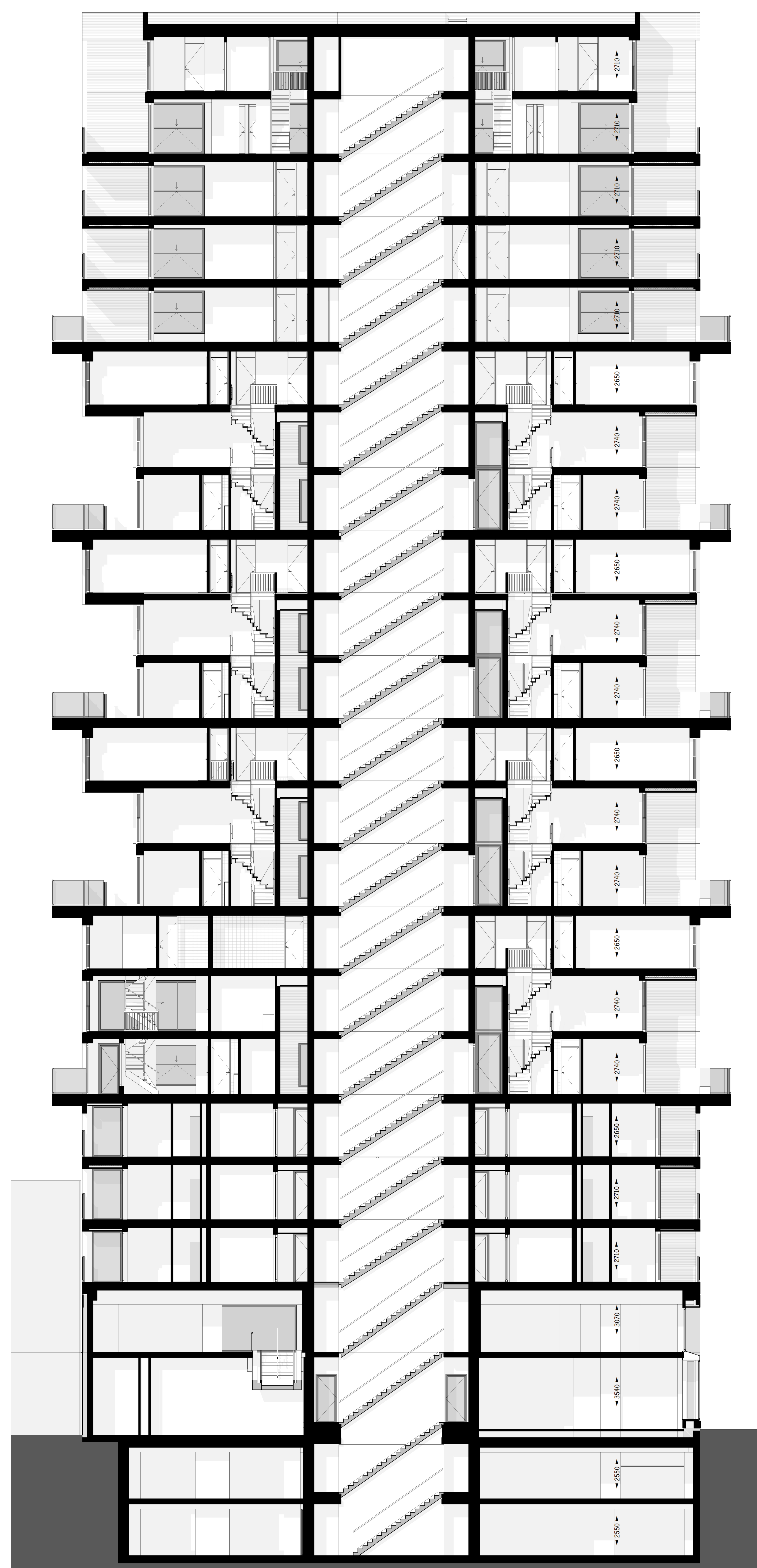
Doorsnede B-B 1:100
