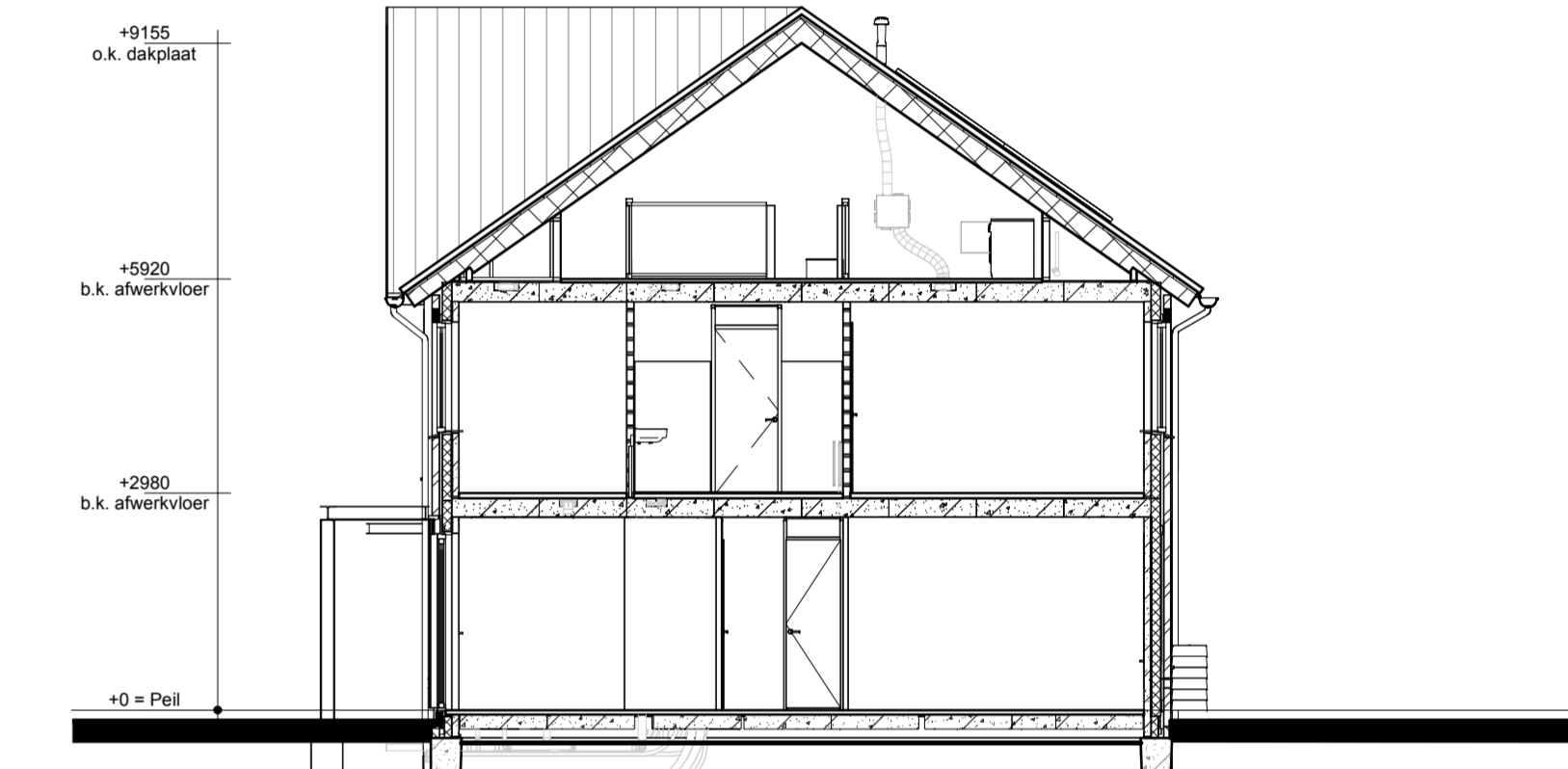
Doorsnede A-A
